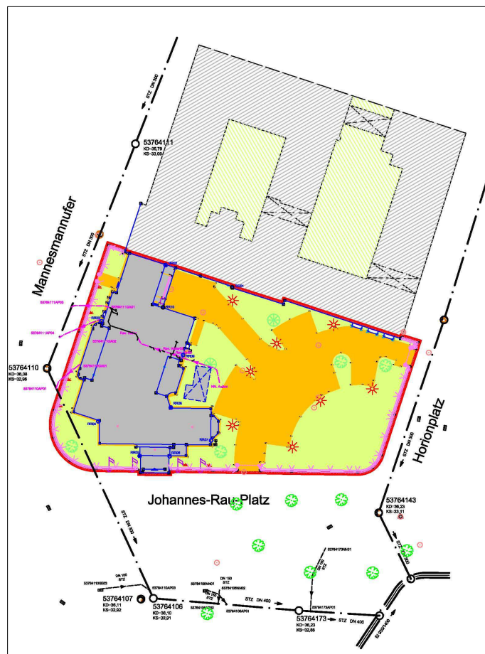
Lageplan Bestand
